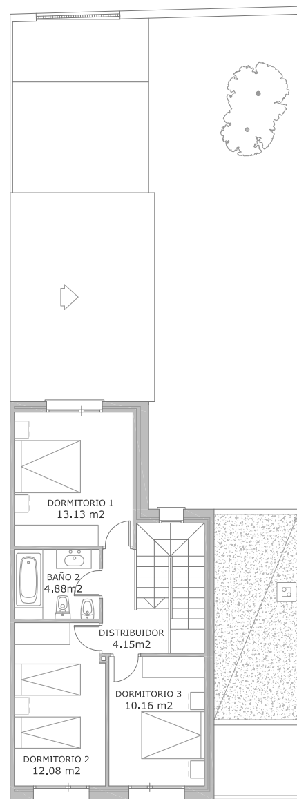
PLANTA PRIMERA
