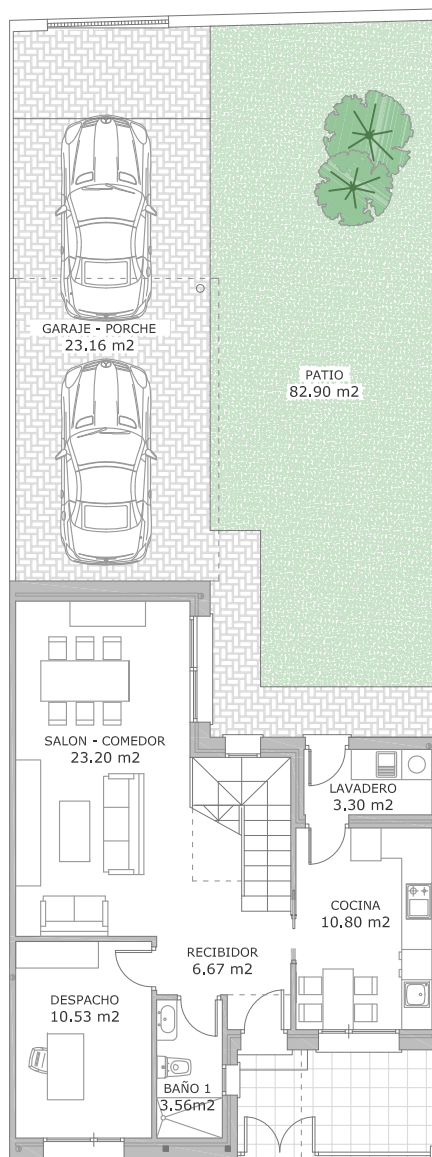
PLANTA BAJA
